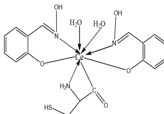
[Ce(BO) 2 (L 4 ).2H 2 O]
