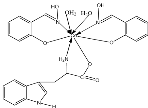
[Ce(BO) 2 (L 1 ).2H 2 O]
