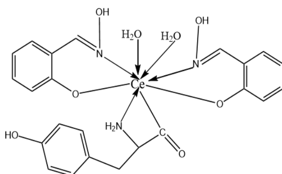
[Ce(BO) 2 (L 3 ).2H 2 O]
