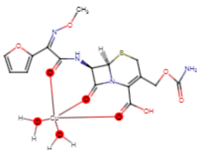
Cu Complex
